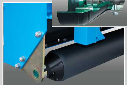
Rullo d'appoggio con fondelli smontabili, labirinti e guarnizioni su cuscinetti lubrificati a vita. Roller with removable ends, labyrinths and seals on life-greased bearings Rodillo de apoyo con componentes desmontables, laberintos y juntas en rodamientos engrasados de por vida
