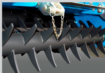
Pick-up anteriore per il sollevamento dei soli sarmenti e il convogliamento in camera di triturazione Front pick-up for lifting the pruning residues and further delivery into the mulching chamber Dispositivo de recogida (pick-up) frontal para levantar los restos de poda y llevarlos a la cámara de trituración
