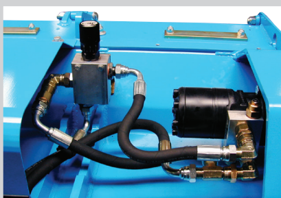
Trasmissione idraulica del pick-up con valvola di regolazione di velocità e possibilità di invertire il moto Pick-up hydraulic drive with speed regulation valve and possibility to reverse the direction of rotation Transmisión hidráulica del dispositivo de recogida (pick-up) con válvula de regulación de velocidad y posibilidad de invertir el sentido de rotación
