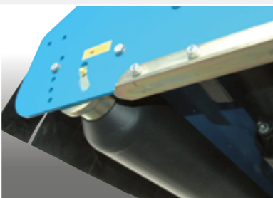
Rullo Ø 140 mm a fondelli fissi regolabile in 5 posizioni Roller: Ø 140 mm with fixed ends adjustable in 5 positions Rodillo: Ø 140 mm con extremos fijos en 5 posiciones
