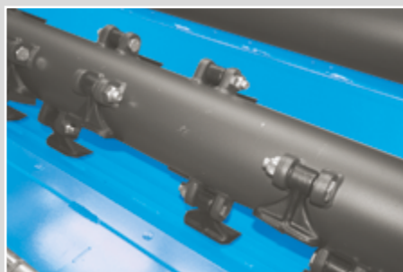
Equilibratura elettronica ai massimi regimi di lavoro della macchina. Coltelli e mazze su perno trattato Ø 20 mm per una minore usura.
